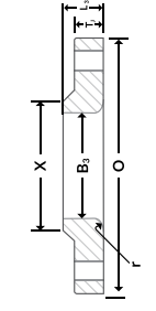
Brida traslape
