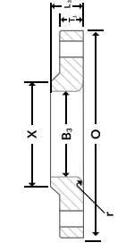
Brida traslape
