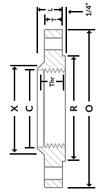
Brida roscada
