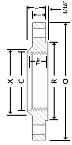
Brida roscada
