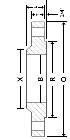
Brida deslizable
